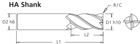
HA Shank
